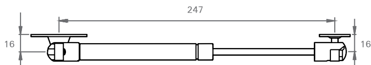
מחבר לדלת
