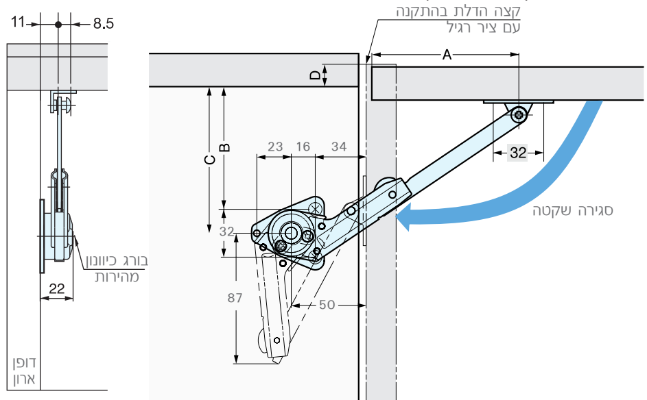
זרוע לדלת מתרוממת
