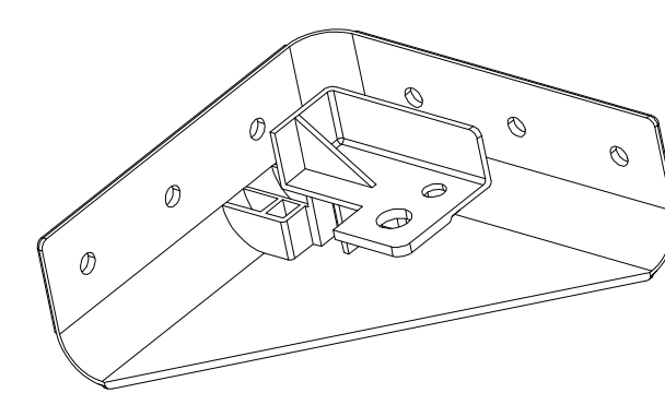
F35-C28 x1
