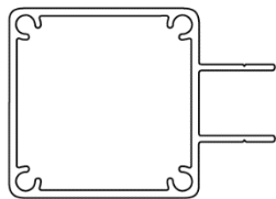
עמוד גדר חד כיווני 2 X 58 X 58 מ"מ
