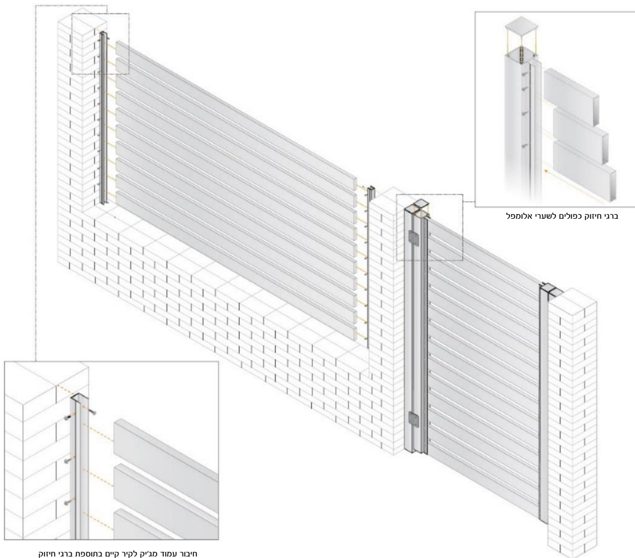
חיבור עמוד מג"ק לקיר קיים בתוספת ברגי חיזוק
