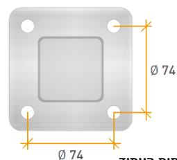
לוח בסיס העמוד
