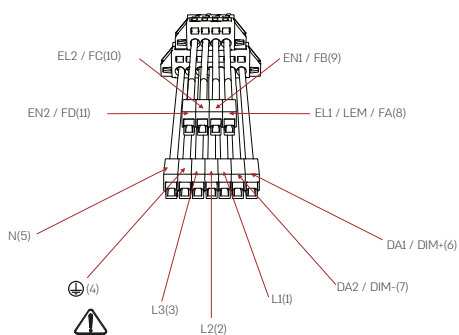
11 חוטים, 9 פינים
