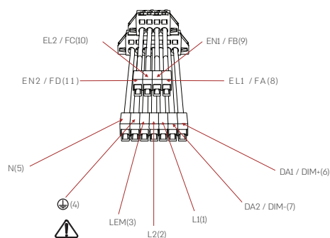
11 חוטים, 10 פינים
