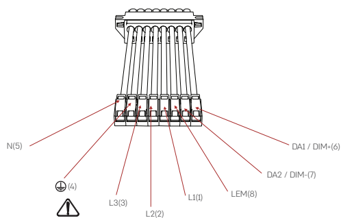
8 חוטים, 6 פינים
