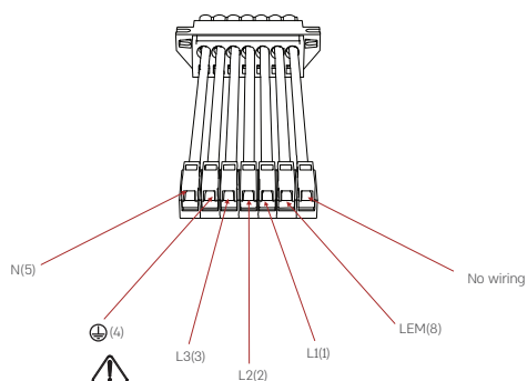
6 חוטים, 4 פינים
