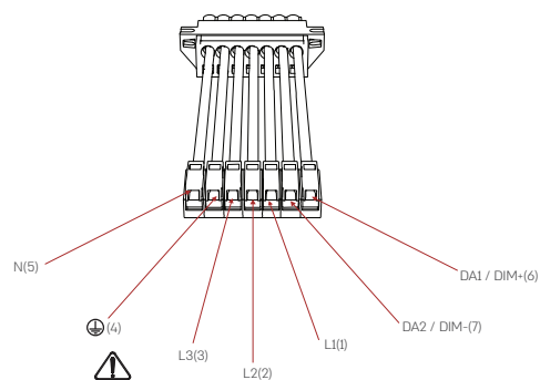
7 חוטים, 5 פינים
