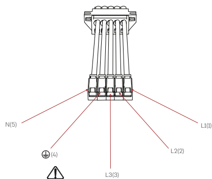
5 חוטים, 3 פינים
