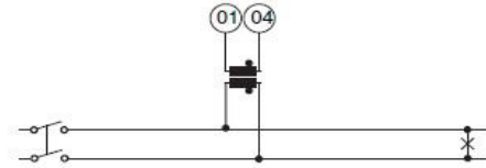
חיבור עם שנאי מתח
